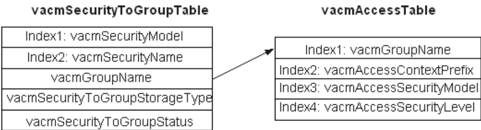
图 190-1 vacmSecurityToGroupTable 表与 vacmAccessTable 表之间的关系
